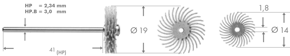
Акриловый диск со встроенными абразивами
